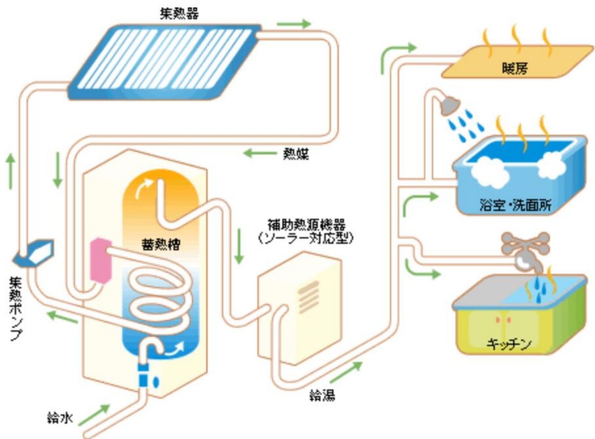
住宅用太陽熱利用システム（出典：環境省）
